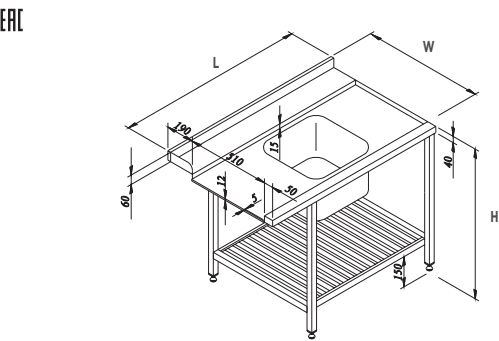
Dishwasher Inlet Table With Under Shelf Table d'entrée Lave-vaisselle Avec Une Étagère Basse Ajourée
