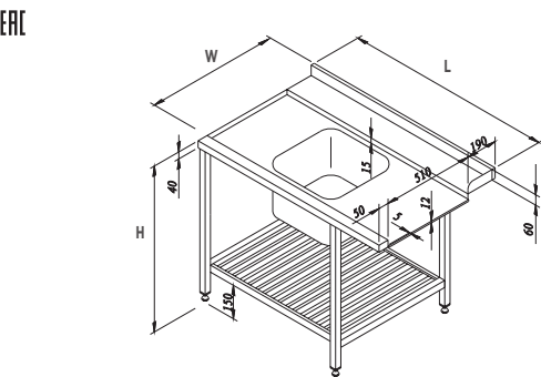
Dishwasher Inlet Table With Under Shelf Table d'entrée Lave-vaisselle Avec Une Étagère Basse Ajourée
