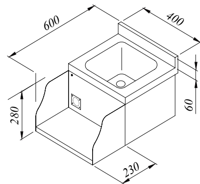
Blender Bench Counter Top Stand de Blender à Poser
