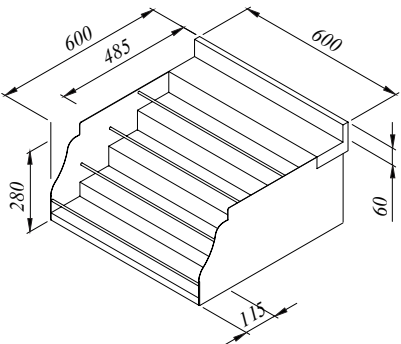
Bottle Display Counter Top Présentoir a Bouteilles a Poser
