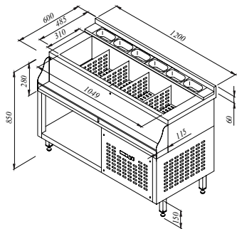
Refrigerated Cocktail Preparation Unit Table de Préparation a Cocktails Réfrigérée
