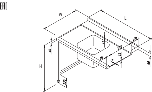
Dishwasher Inlet Table Table de d'entrée Lave-vaisselle
