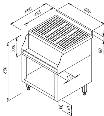
Bar Bench With Drainer And Bottle Display Table De Bar Avec Égouttoir Et Présentoir À Bouteilles
