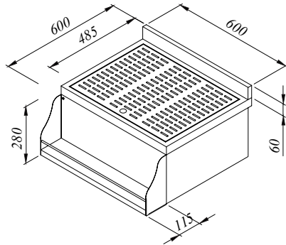
Bar Bench With Drainer & Bottle Display Counter Top Table de Bar Avec Égouttoir & Présentoir a Bouteilles a Poser
