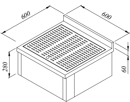
Bar Bench With Drainer Counter Top Table de Bar Avec Égouttoir a Poser
