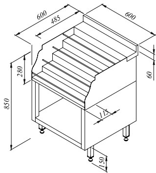
Bottle Display Présentoir À Bouteilles
